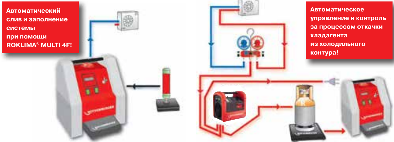
Применение ROKLIMA MULTI 4F (слив и заполнение)
